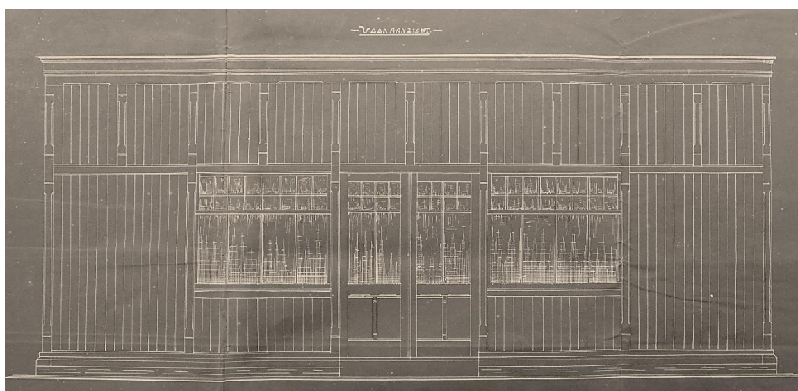
Voorraanzicht
